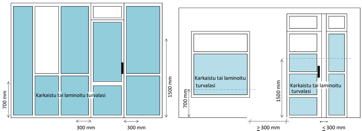
Kuva 2. Ikkuna- ja ovilasirakenteet muualla kuin asunnossa (ei putoamisvaaraa)
