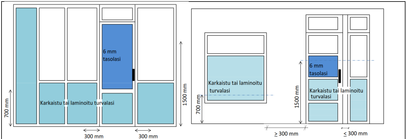
Kuva 1. Ikkuna- ja ovilasirakenteet asunnossa (ei putoamisvaaraa)
